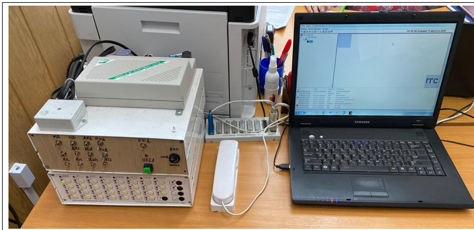
Система диспетчерского контроля за эксплуатацией лифтов типа «Обь»
