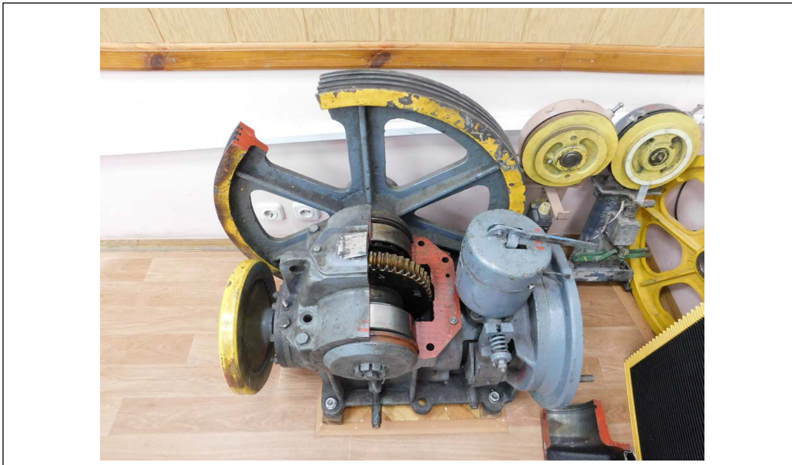
Лебедка пассажирского лифта в разрезе
